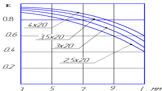
12-сурет. Қоспа бөлшектерінің ұзындығына қатысты төртбұрыш пішінде тесіктері бар електерден бұрыштап өту ықтималдылығының графигі
