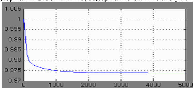
Рисунок 7 - График изменения содержания Cu в шлаке при изменении содержания SiO_2 в шихте
