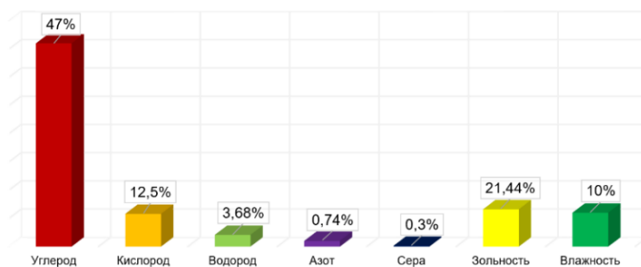
Рисунок 2 – Элементарный состав угля разреза Каражыра
