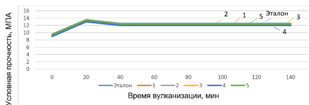
Рисунок 1 – Зависимость условной прочности от времени вулканизации
