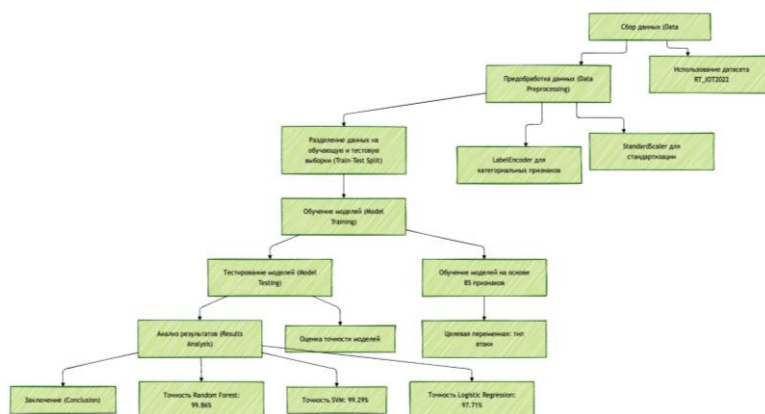
Рисунок 1 – Блок-схема процесса классификации данных
