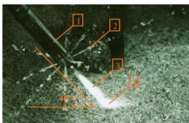
Рисунок 6 – Взаимодействие детонационного факела 3 с гранитной поверхностью 4
