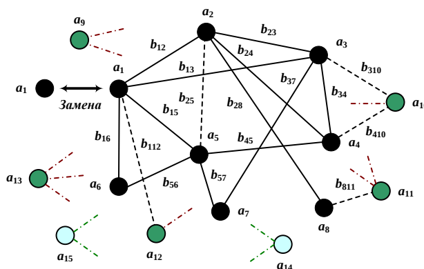
Рисунок 2 – Модель фрагмента МСС в виде неориентированного графа
