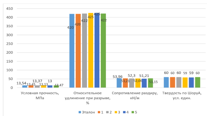
Рисунок 5 – Диаграмма зависимости физико-механических свойств резины для изготовления уплотнений гидрозатворов от содержания ОЧН и цеолита
