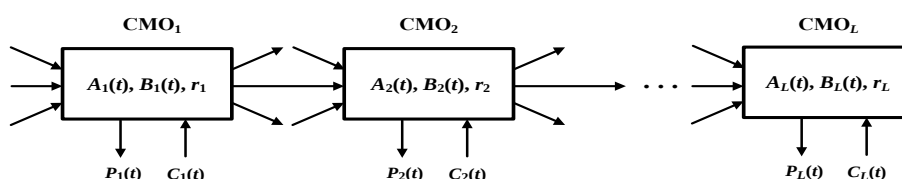
Рисунок 1 – Модель тракта обмена информацией в виде многофазной СМО
