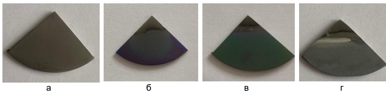
Рисунок 2 – Образцы до и после МДО а) исходный; б) № 1; в) № 2; г) № 3
