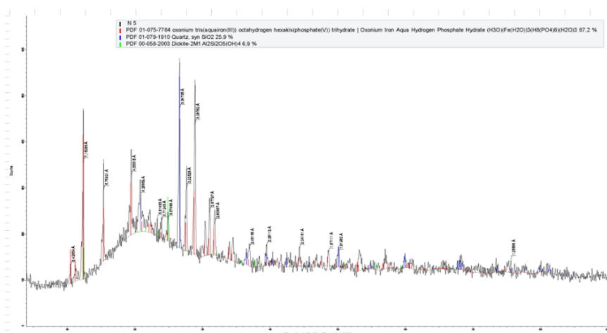
Рисунок 1 – Рентгенограмма нерастворимого остатка
