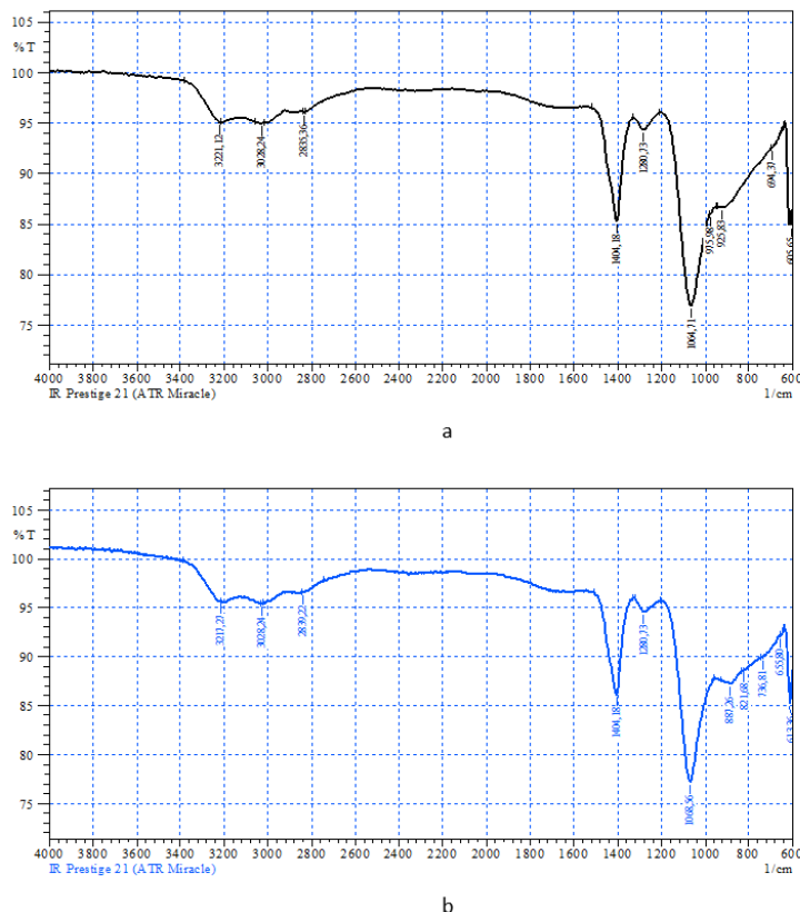
Рисунок 4 – ИК-спектры образцов сульфоаммофоса: а – 2, б – 3.
