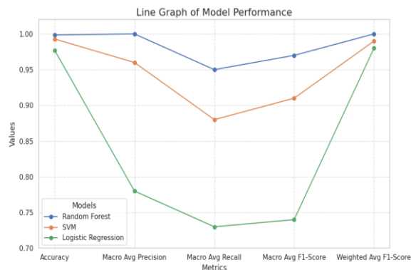
Рисунок 3 – Линейный график для каждой модели
