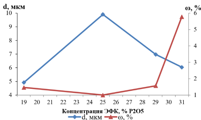
Рисунок 5 – Зависимость размера кристаллов и влажности сульфоаммофоса от концентрации раствора ЭФК
