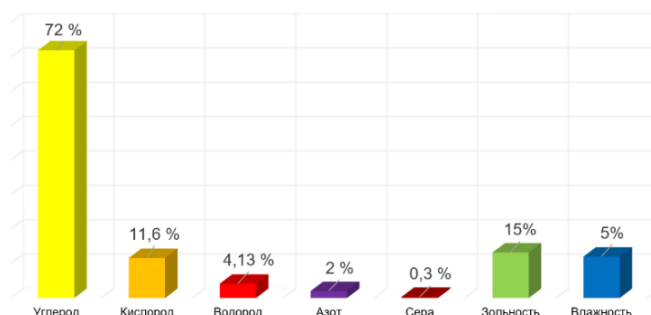
Рисунок 3 – Элементарный состав Кузнецкого угля
