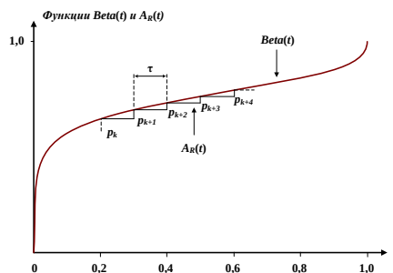
Рисунок 3 – Аппроксимация бета-распределения функцией A_R(t)
