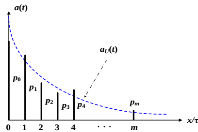
Рисунок 2 – Замена гистограммы a(t) непрерывной функцией a_U(t)
