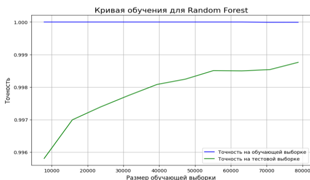
Рисунок 7 – Кривая обучения
