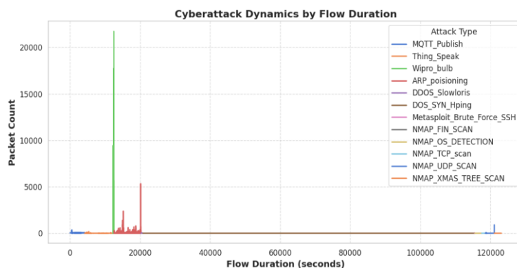
Рисунок 4 – Динамика кибератак по продолжительности потока
