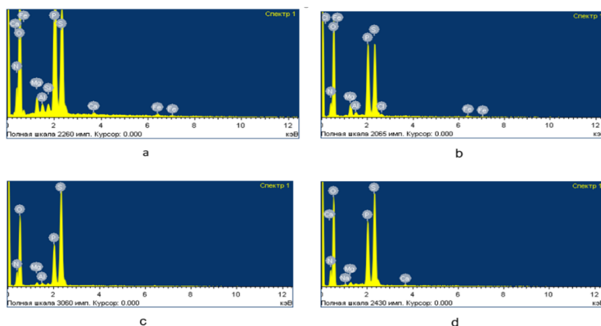
Рисунок 3 – Спектрограмма образцов сульфоаммофоса: а – 1, б – 2, с – 3, d – 4
