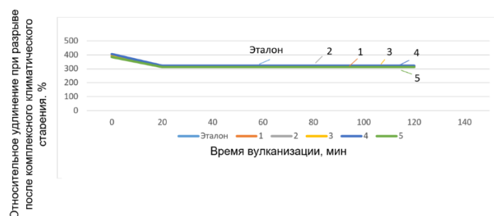
Рисунок 4 – Зависимость относительного удлинения при разрыве после комплексного климатического старения
