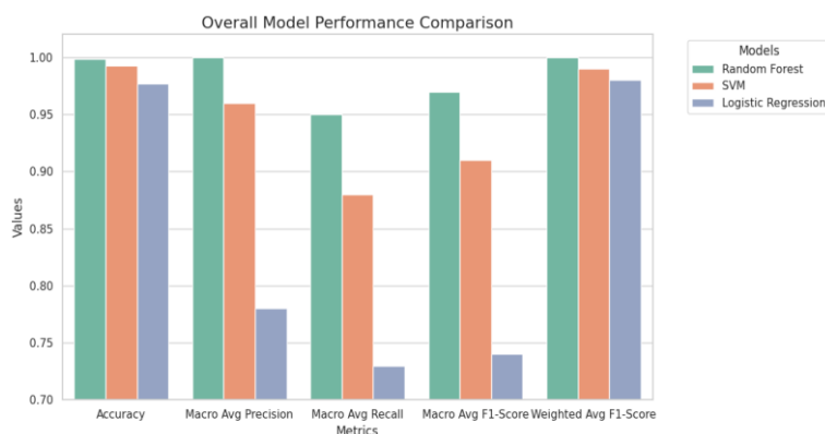
Рисунок 2 – Общий сравнительный анализ производительности моделей
