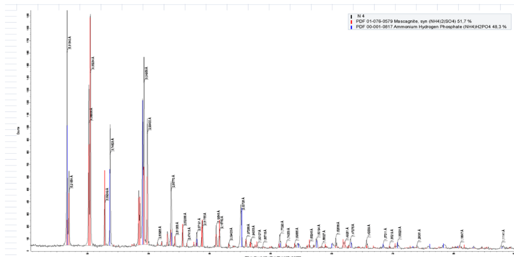
Рисунок 6 – Рентгенограмма сульфаммофоса, полученного в оптимальных условиях
