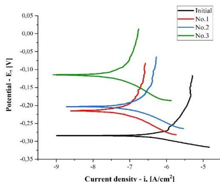
Рисунок 4 – Поляризационные кривые титана до и после МДО
