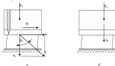
Сурет 3 – Кесу режимдерінің сұлбасы
