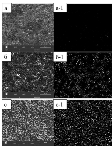
Рисунок 3 – СЭМ снимки образцов после МДО а) № 1; б) № 2; с) № 3 Пористость покрытий: а – 1) № 1; б – 1) № 2; с – 1) № 3
