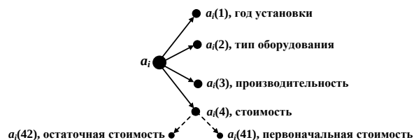
Рисунок 3 – Сущность элементов графа на примере вершины a_i
