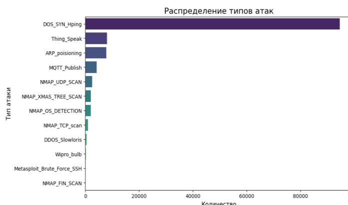
Рисунок 8 – Распределение типов атак
