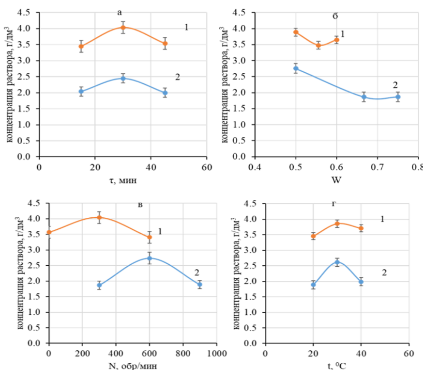
Рисунок 1 – Частные зависимости изменения общего содержания органической и минеральной части донных отложений от массовой доли отложений (а), времени перемешивания смеси (б), скорости перемешивания (в) и температуры (г)
