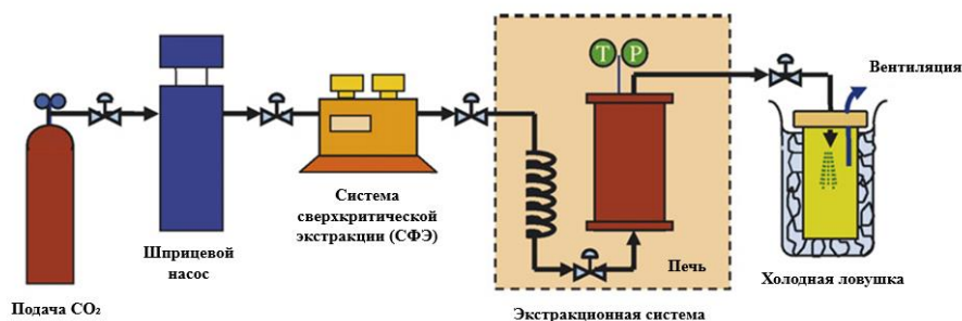
Рисунок 2 – Схема установки для сверхкритической флюидной экстракции [15]
