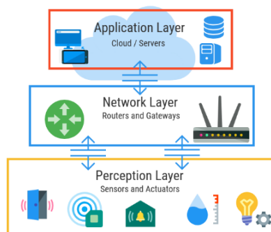
Сурет 1 – IoT архитектурасы
