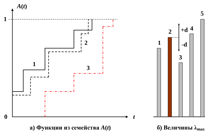
Рисунок 5 – Примеры устойчивости для функций A(t) и пиковых значений \lambda
