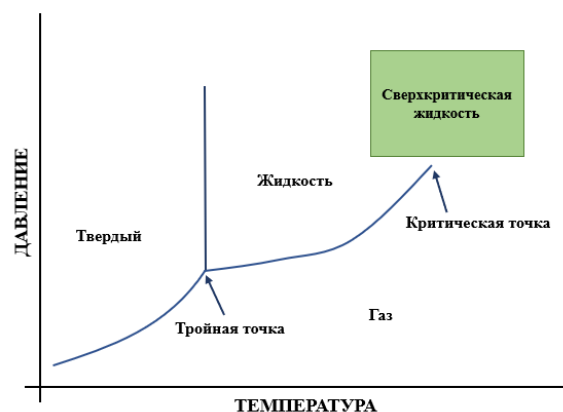
Рисунок 1 – График образования сверхкритической жидкости [1]
