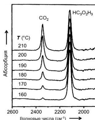
Рисунок 5 – ИК-спектры пропускания для декарбоксилирования 0,5 моляльной пропиоловой кислоты в зависимости от температуры и давления [64].
