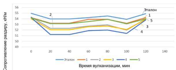
Рисунок 3 – Зависимость сопротивления раздиру от времени вулканизации
